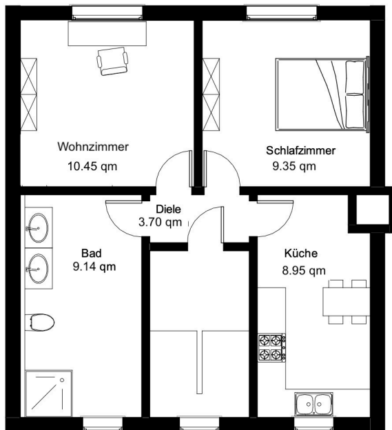
Grundriss DG
